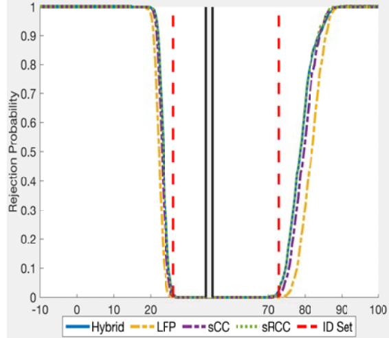
(d) 4 Parameters, 38 Moments
